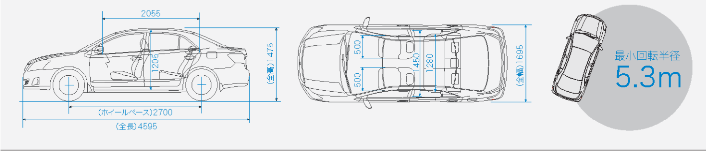
寸法図(単位:mm) 1.8X(2WD)
