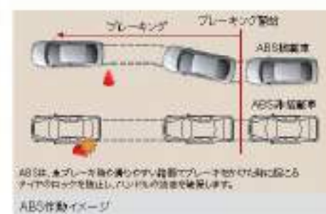
ABS作動イメージ
